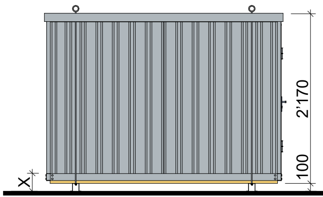
Ansicht A
