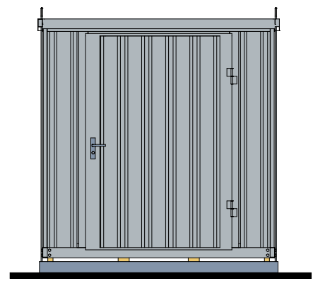
Ansicht B
