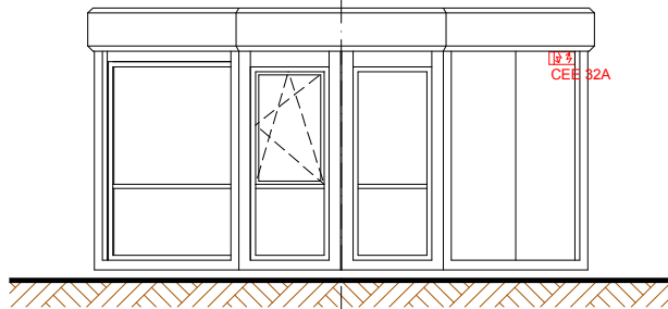
Ansicht B
