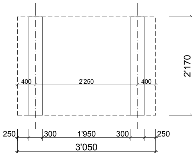
Vue A
