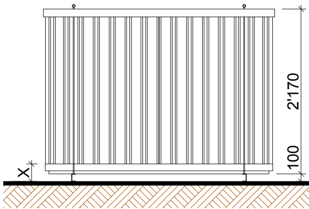
Vue A
