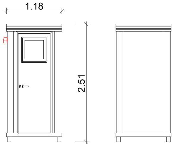
Ansicht A
