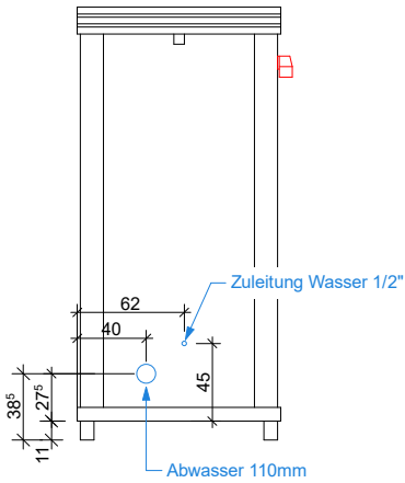
Ansicht C
